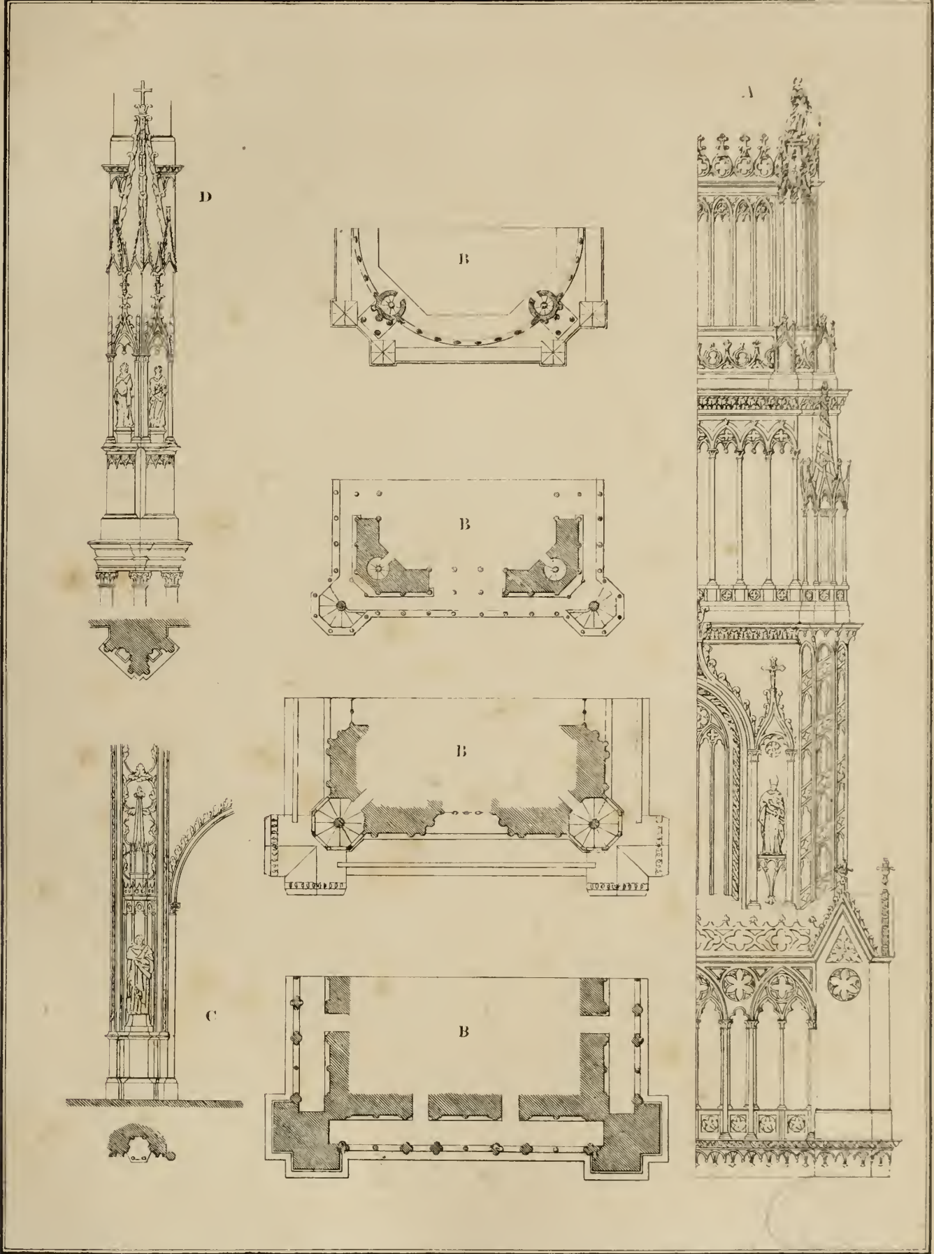
A, détails de la tour. B,B,B,B, plans des divers étages de la tour. C, porte du milieu. D, partie supérieure des contreforts de la façade
